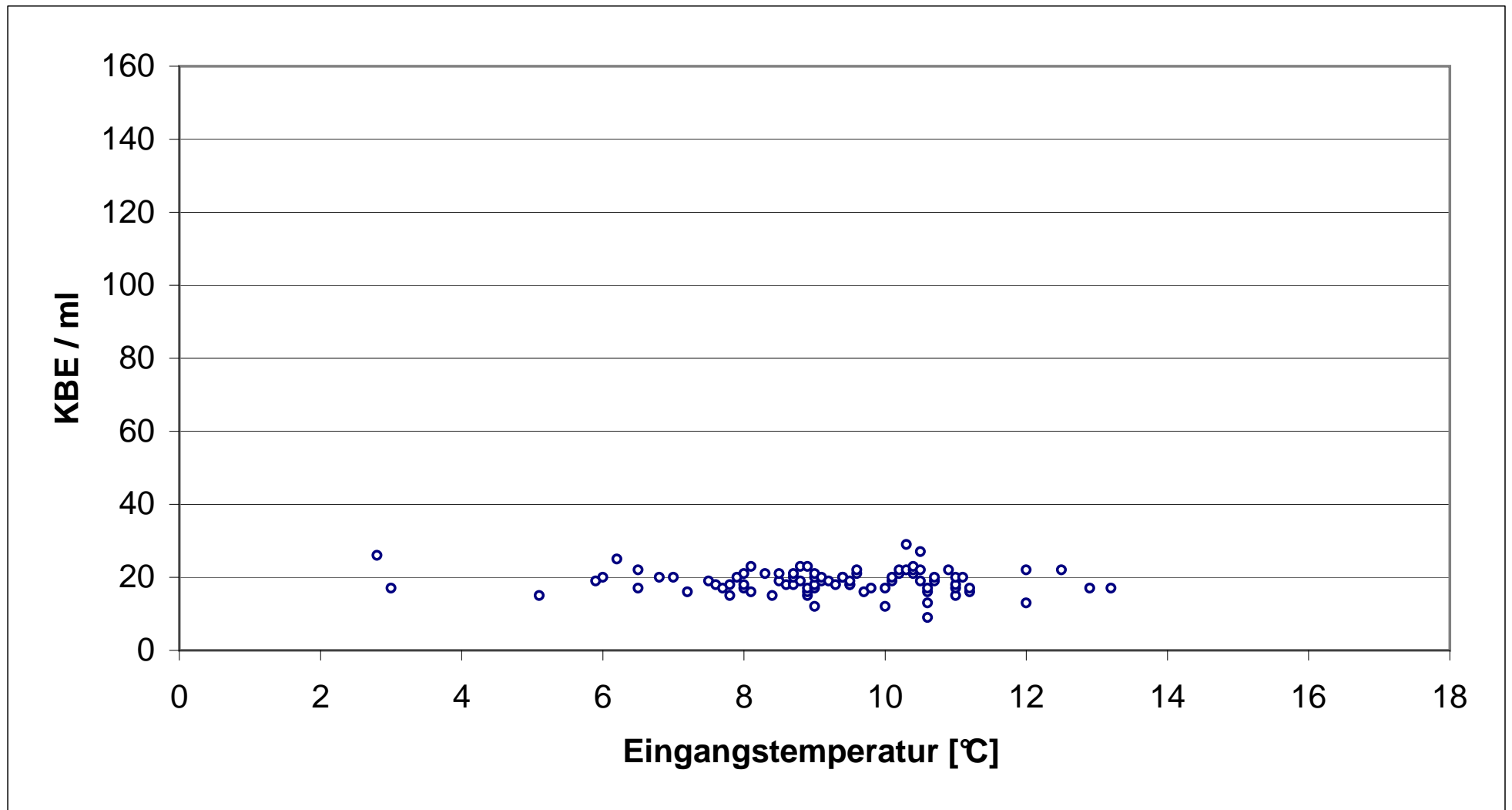
Abb. 14 Koloniezahlen bei 20°C ( AF Gruppe A) in Abhängigkeit von der Eingangstemperatur
