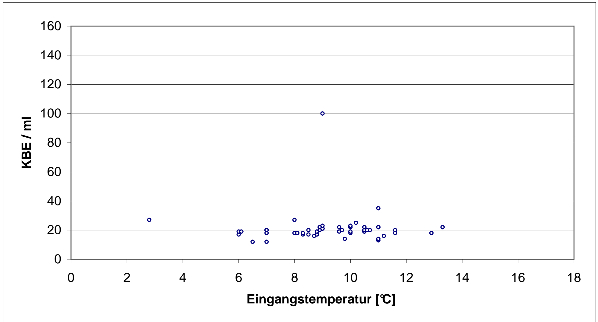
Abb. 16 Koloniezahlen bei 36°C ( NF Gruppe A) in Abhängigkeit von der Eingangstemperatur
