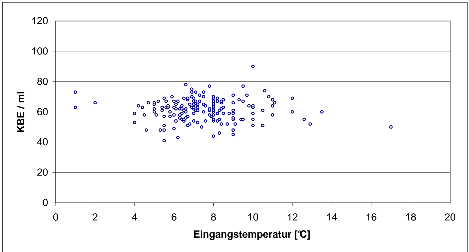
Abb. 15 Koloniezahlen 36°C [TrinkwV 2001 Anl.5 I d) bb) - Gruppe A] in Abhängigkeit von der Eingangstemperatur
