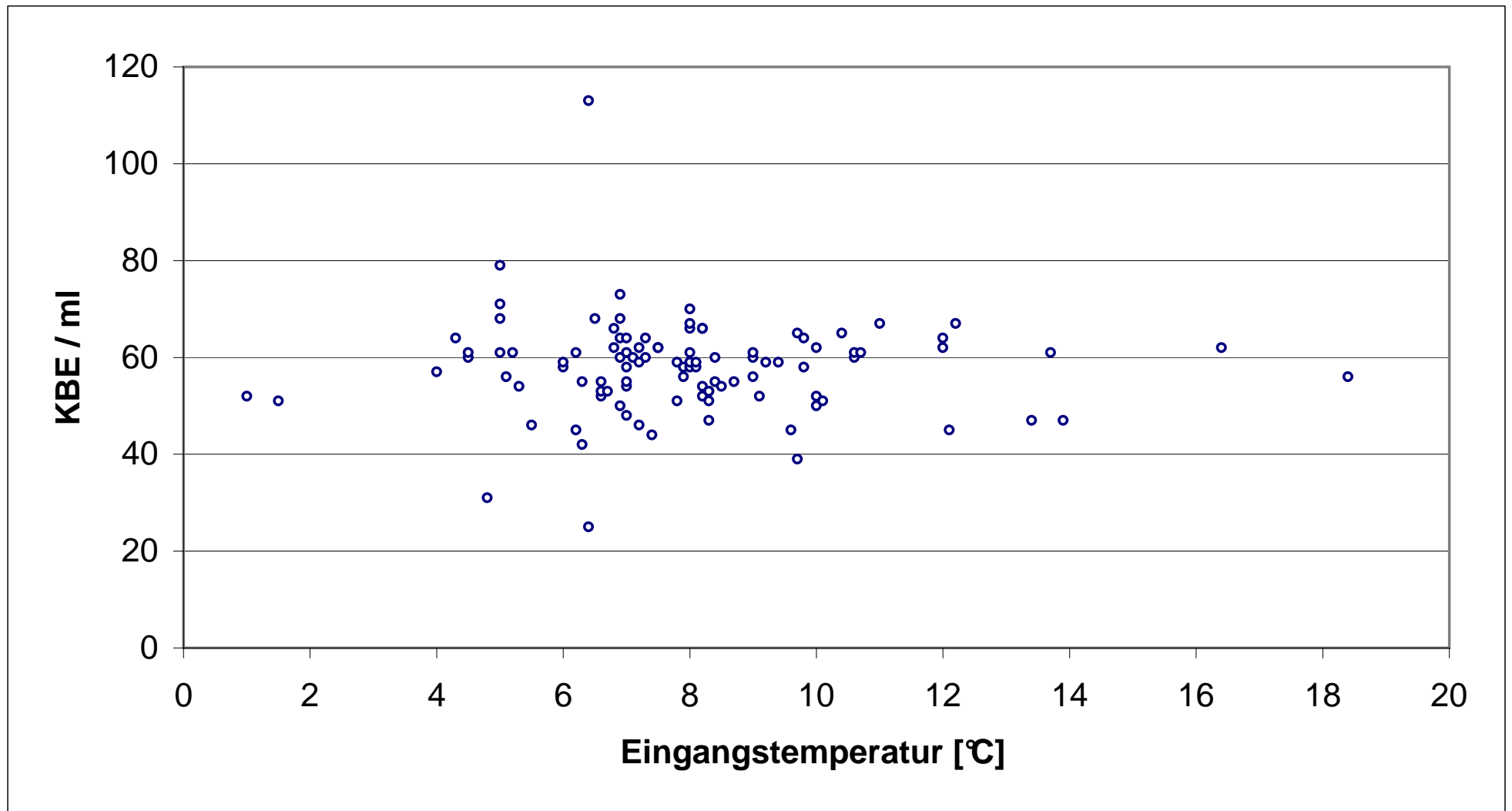
Abb. 18 Koloniezahlen 22°C ( DIN 6222 - Gruppe A) in Abhängigkeit von der Eingangstemperatur
