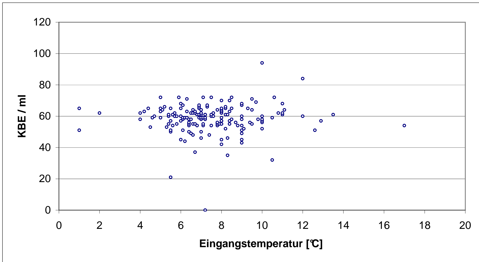
Abb. 14 Koloniezahlen 22°C [TrinkwV 2001 Anl.5 I d) bb) - Gruppe A] in Abhängigkeit von der Eingangstemperatur
