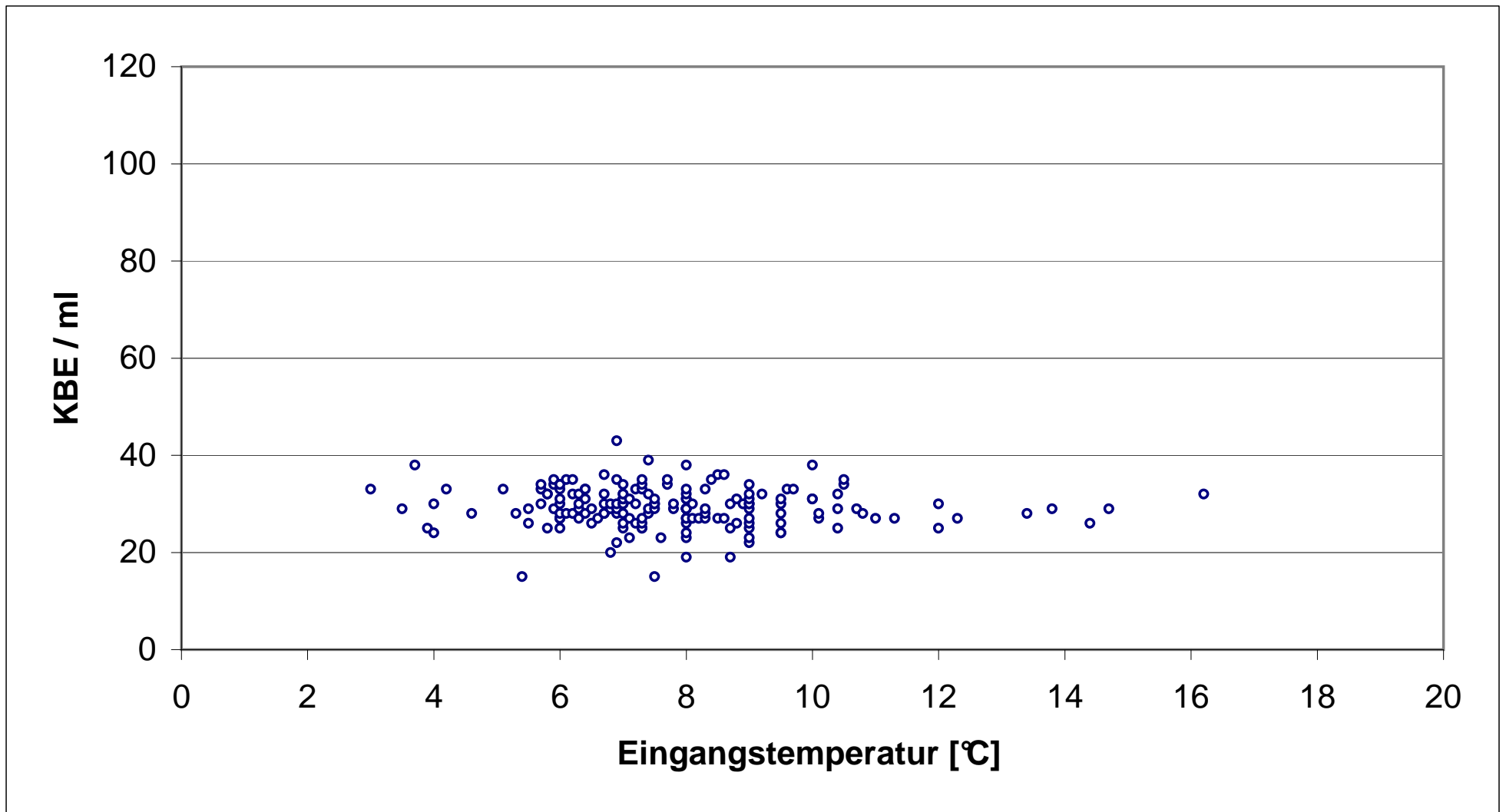
Abb. 16 Koloniezahlen 22°C [TrinkwV 2001 Anl.5 I d) bb) - Gruppe B] in Abhängigkeit von der Eingangstemperatur
