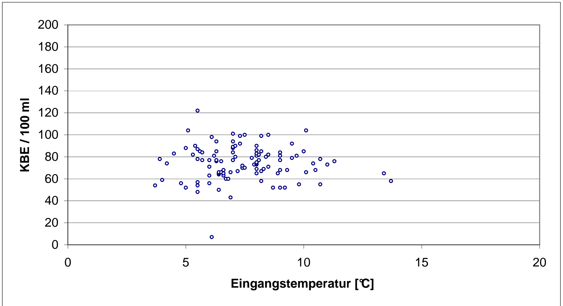
Abb. 9 KBE (Enterokokken Gruppe C) in Abhängigkeit von der Eingangstemperatur
