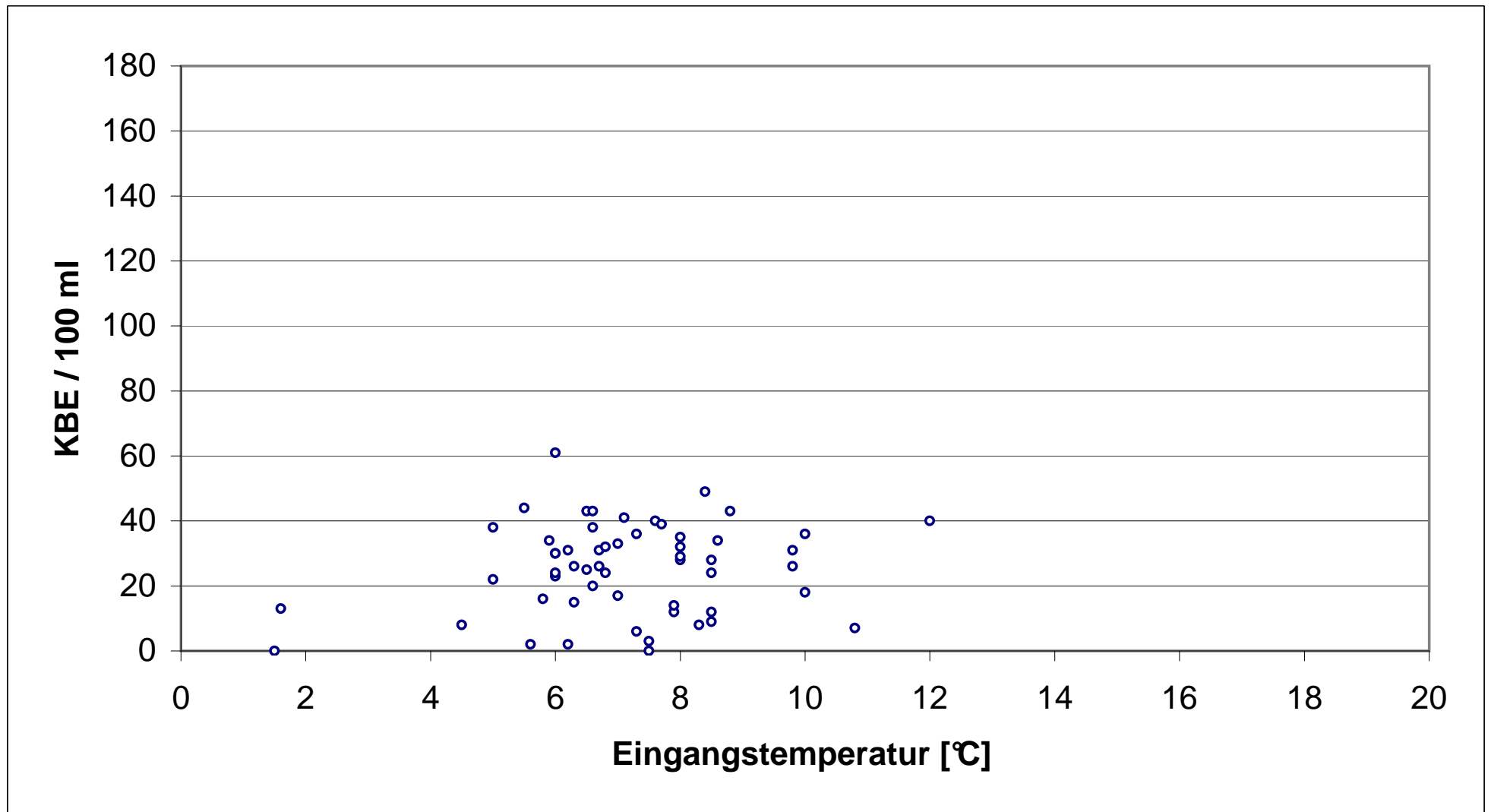
Abb. 11 KBE ( C. perfringens Gruppe A) in Abhängigkeit von der Eingangstemperatur
