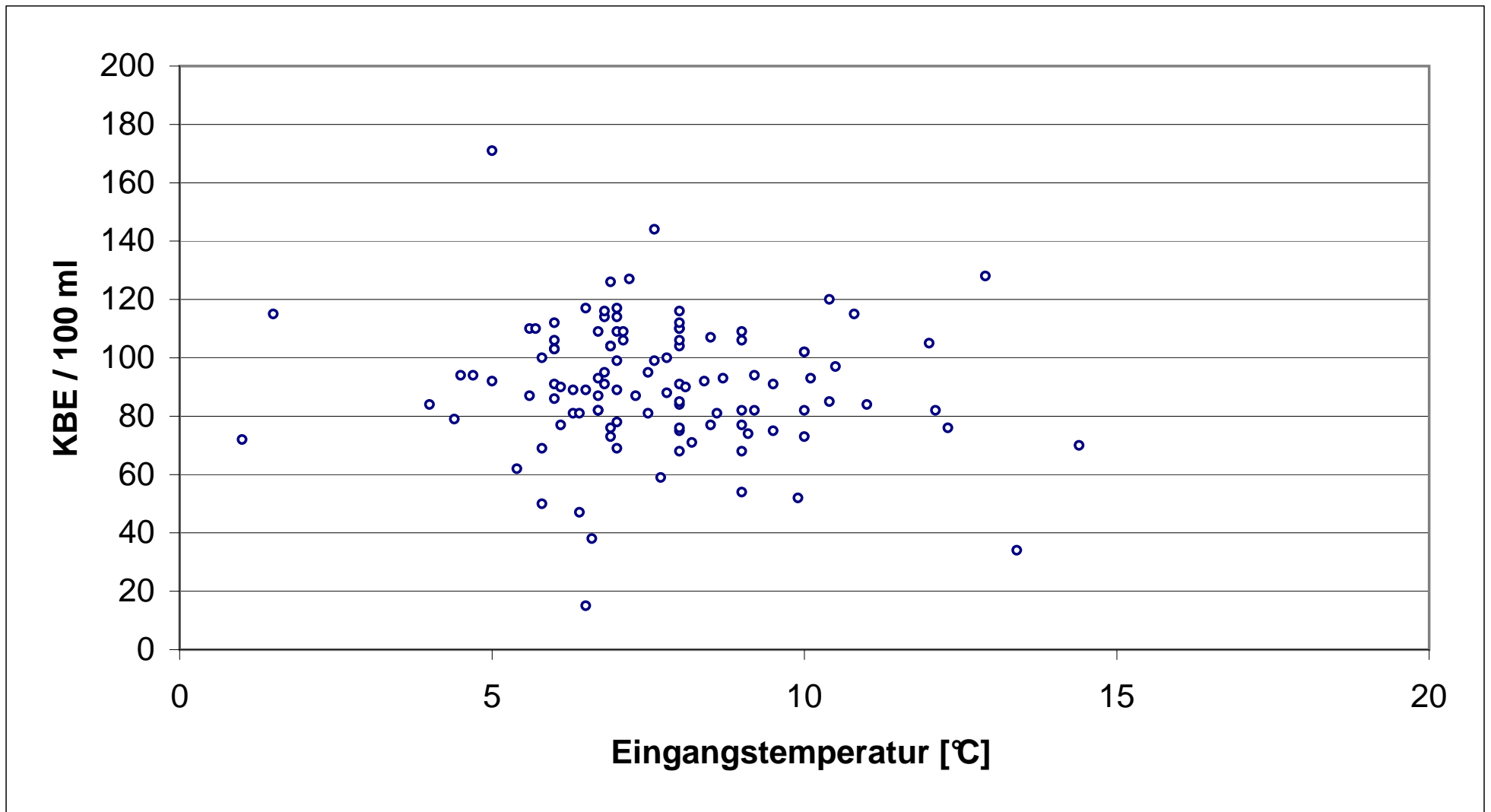
Abb. 8 KBE (Enterokokken Gruppe B) in Abhängigkeit von der Eingangstemperatur
