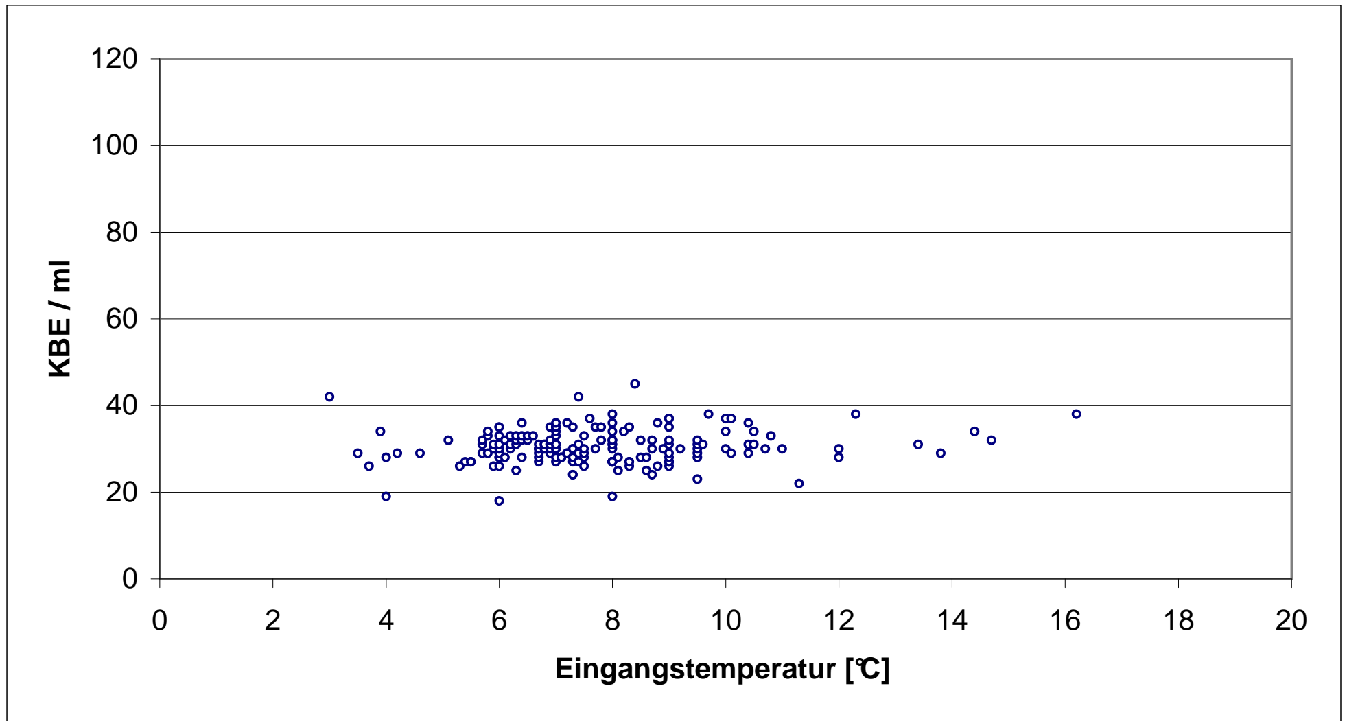
Abb. 17 Koloniezahlen 36°C [TrinkwV 2001 Anl.5 I d) bb) - Gruppe B] in Abhängigkeit von der Eingangstemperatur
