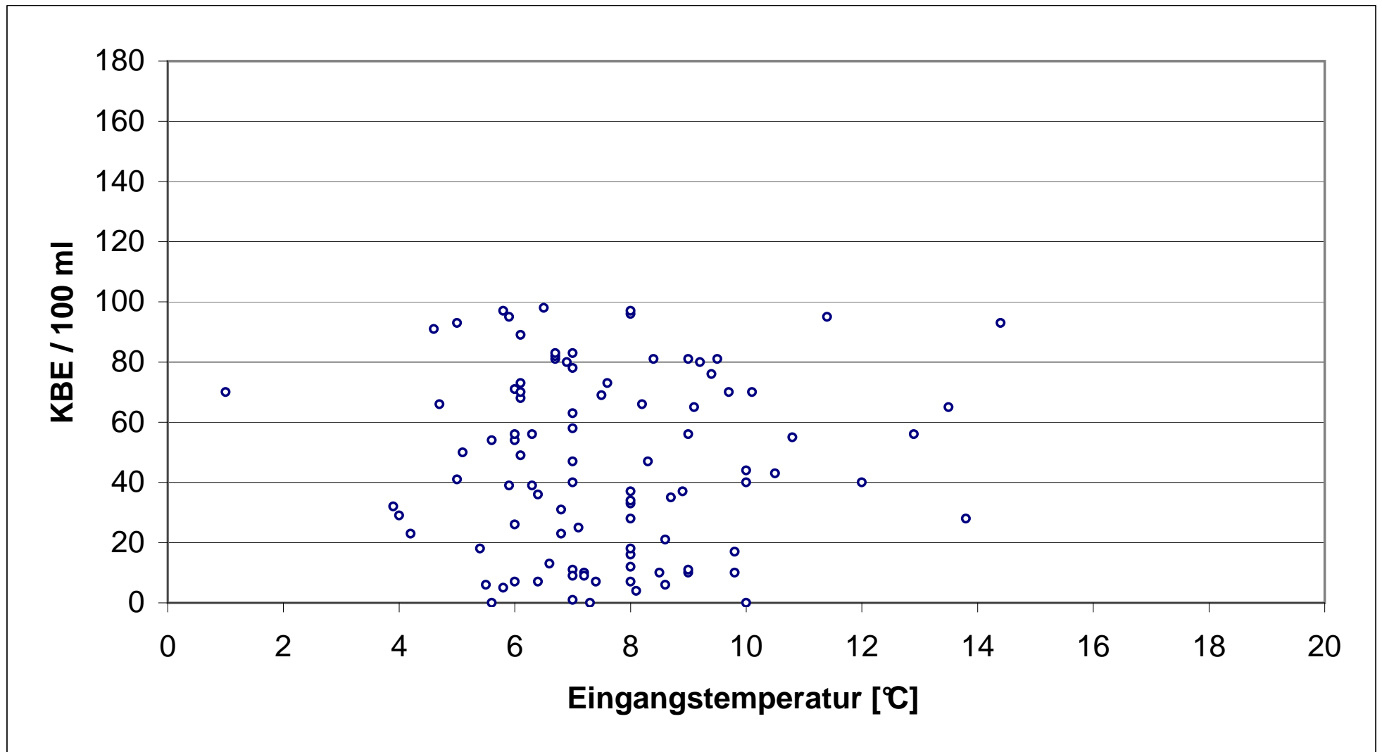
Abb. 12 KBE ( C. perfringens Gruppe B) in Abhängigkeit von der Eingangstemperatur
