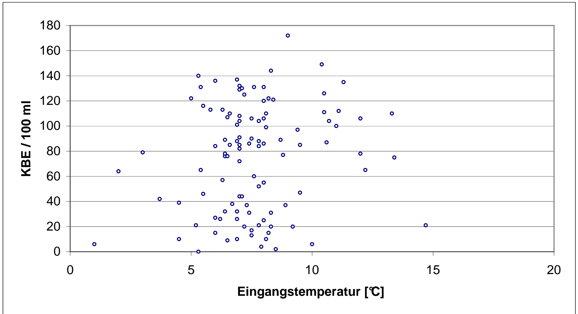
Abb. 13 KBE ( C. perfringens Gruppe D) in Abhängigkeit von der Eingangstemperatur
