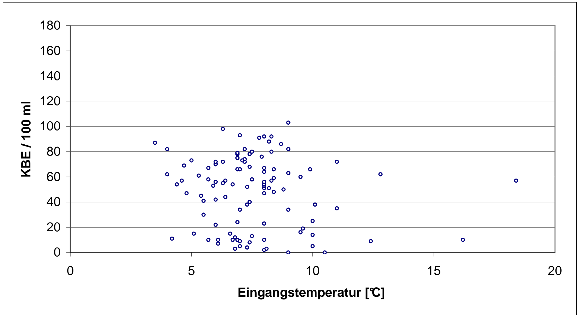
Abb. 13 KBE ( C. perfringens Gruppe C) in Abhängigkeit von der Eingangstemperatur
