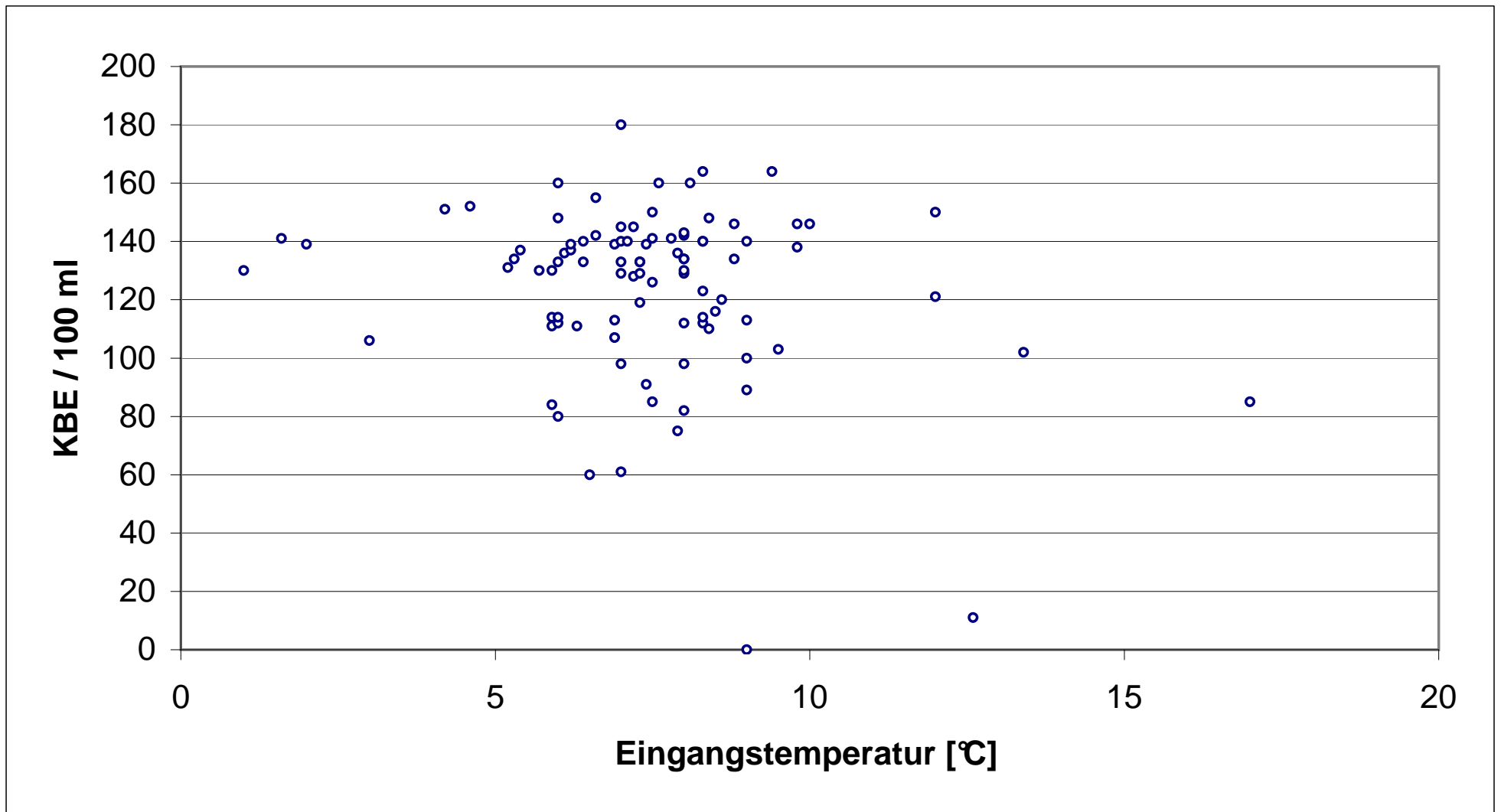
Abb. 7 KBE (Enterokokken Gruppe A) in Abhängigkeit von der Eingangstemperatur
